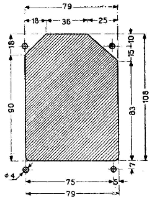
FORATURA TELAIO
